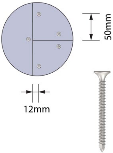
Vis bắn sắt
