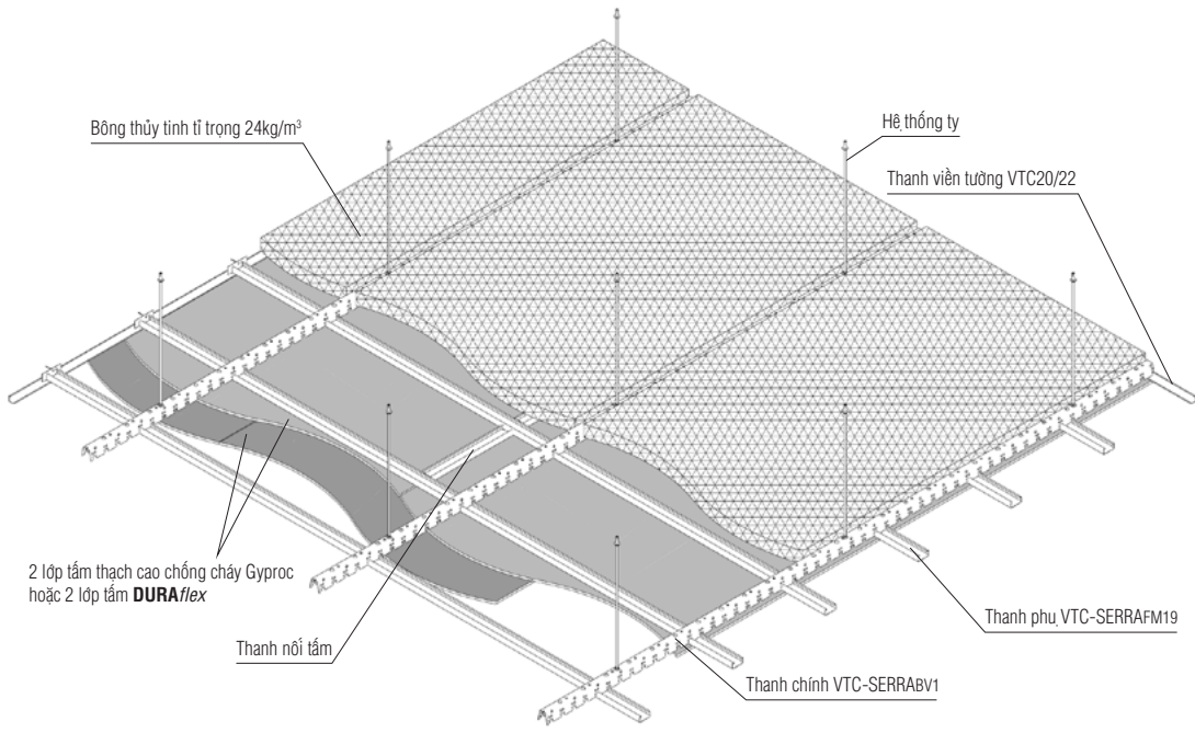
▲ Hệ trần chống cháy sử dụng hệ khung Vinh Tường SERRA, 2 lớp tấm thạch cao chống cháy Gyproc FS và một lớp bông thủy tinh 50mm
