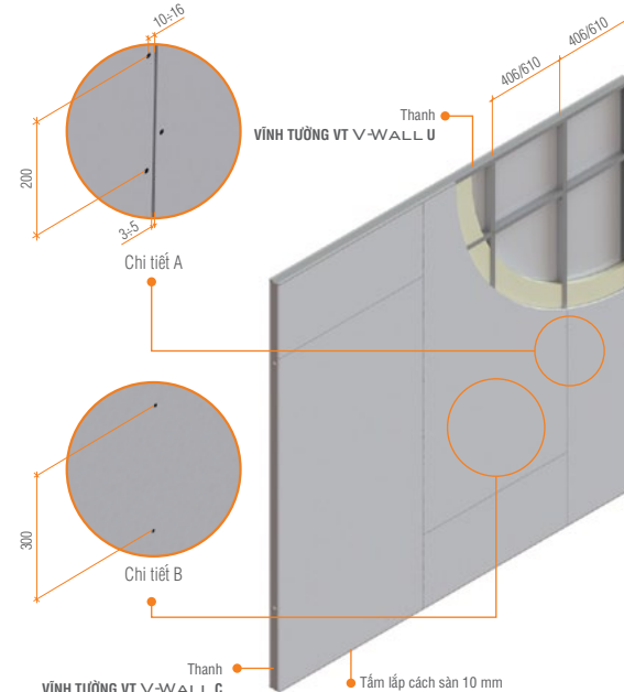
► Hình phối cảnh hệ vách V-Wall
