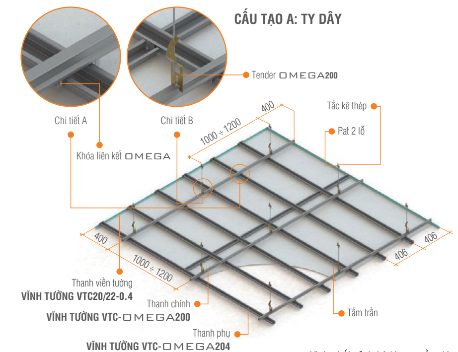
▲ Hình phối cảnh hệ khung trần chìm Vĩnh Tường OMEGA
